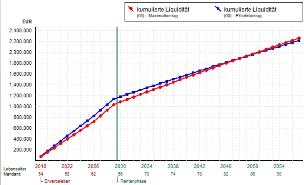
Grafische Break-Even-Analyse
